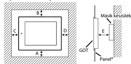
* Panelvastagság: 2,0 – 4,0 mm
