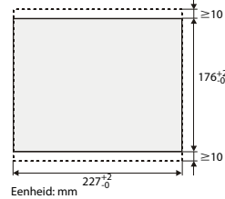
Eenheid: mm
