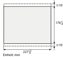
Einheit: mm
