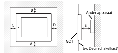
Eenheid: mm
