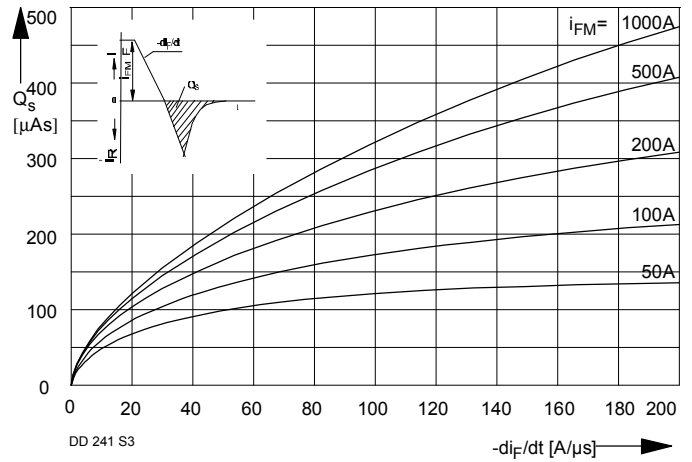
Bild / Fig. 2 Typische Abhängigkeit der oberen Sperrverzögerungsladung Q_s von der abkommutierenden Stromsteilheit -di_F/dt bei t_{vj \max} . Typical relationship between the maximum recovered charge Q_s and the rate of decay of forward current -di_F/dt at t_{vj \max}
