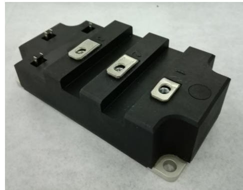
图 2. 模块外形
