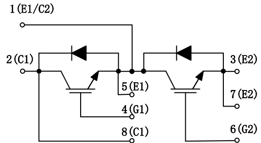
图 1. 电路结构
